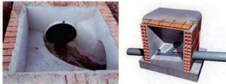
Figura 1 – Fundo das caixas de inspeção
